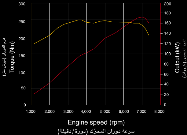
محرك بأربع اسطوانات متقابلة أفقيًا منحنى أداء المحرك Horizontally Opposed 4-cylinders Engine Engine Performance Curve
